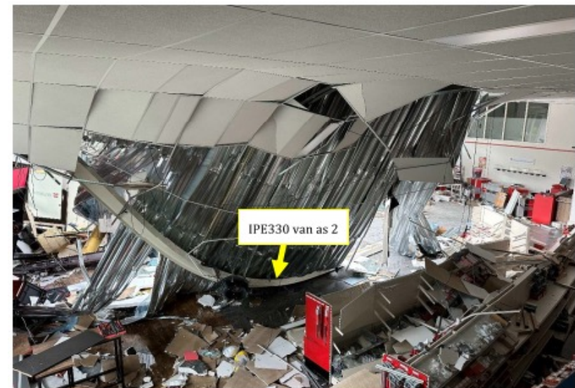
figuur 9 Schade gezien vanuit de binnenzijde van het bedrijfspand.
