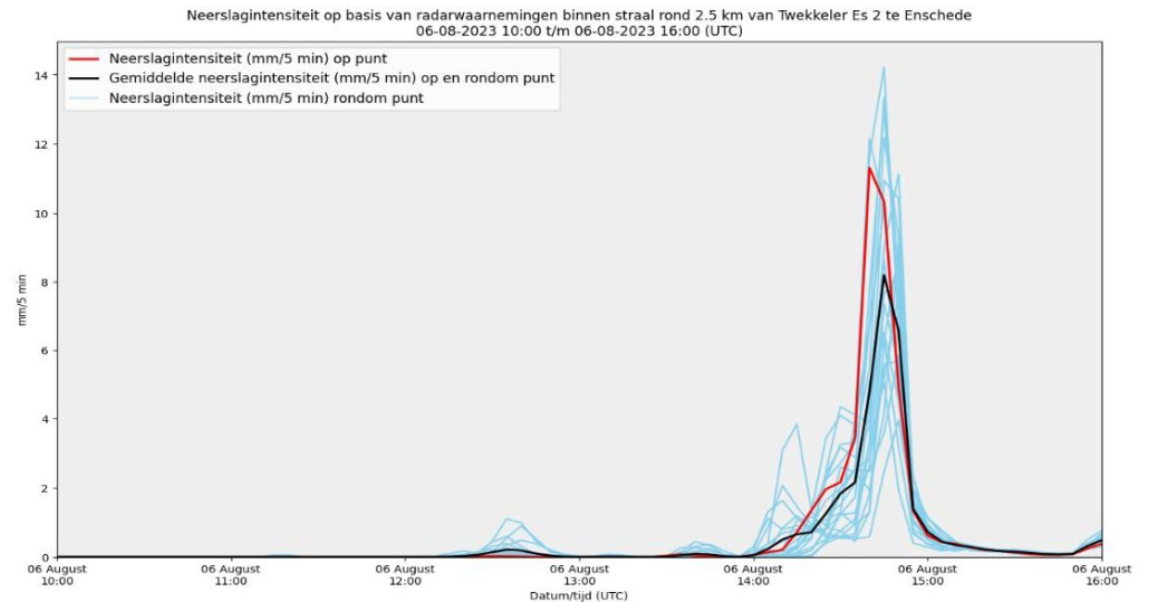
figuur 20 Neerslagintensiteit op en rondom schadelocatie [10].
