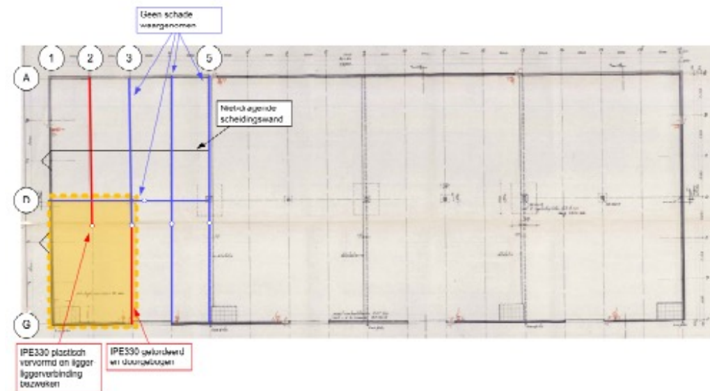
figuur 6 Schadegebied en een deel van de constructie schematisch weergegeven.
