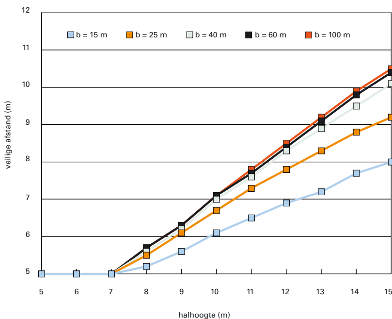
5. De veilige afstand tussen stalen hallen als functie van de hoogte van de hal voor verschillende halbreedten b op basis van NEN 6068 (2004).
