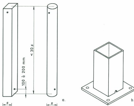
6. Gaten in het buisprofiel voorkomen drukopbouw door waterdamp tijdens brand [3].
