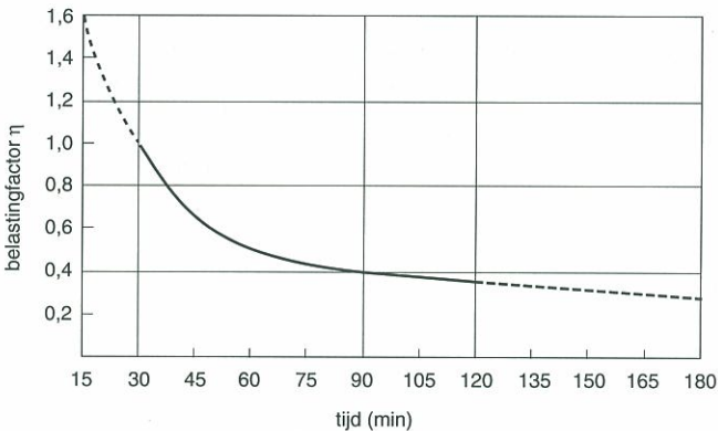
3. Belastingfactor \eta voor ongewapende buiskolommen, afgeleid uit proefresultaten. Tot 90 minuten brandwerendheid is de grafiek een polynoom, daarboven een rechte lijn. Voor brandwerendheden lager dan 30 of hoger dan 120 minuten is geëxtrapoleerd.
