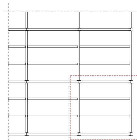
plattegrond staalconstructie van een fictief gebouw
