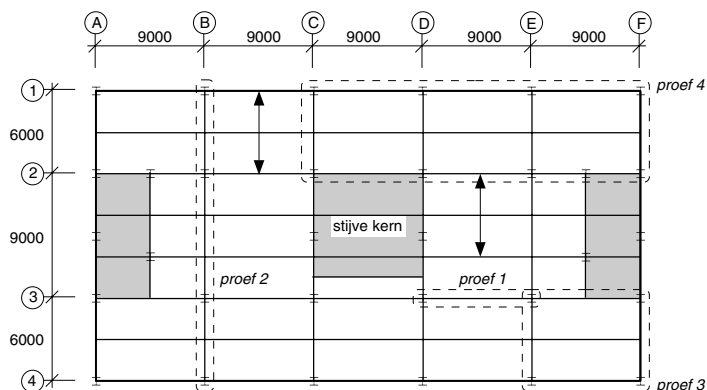
4. Plattegrond van het gebouw, met de plaats en de grootte van de vier brandproeven.
