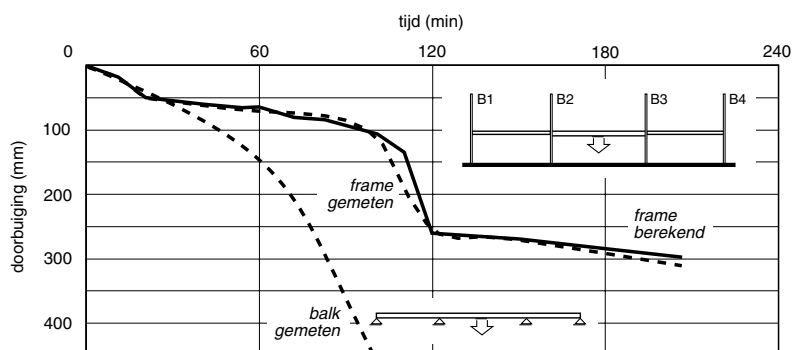
6. Ingekleemde ligger: gemeten en berekende maximale doorbuiging.
