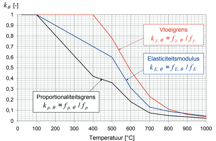
Figuur 1: Reductiefactoren voor de mechanische eigenschappen van staal in functie van de temperatuur.
